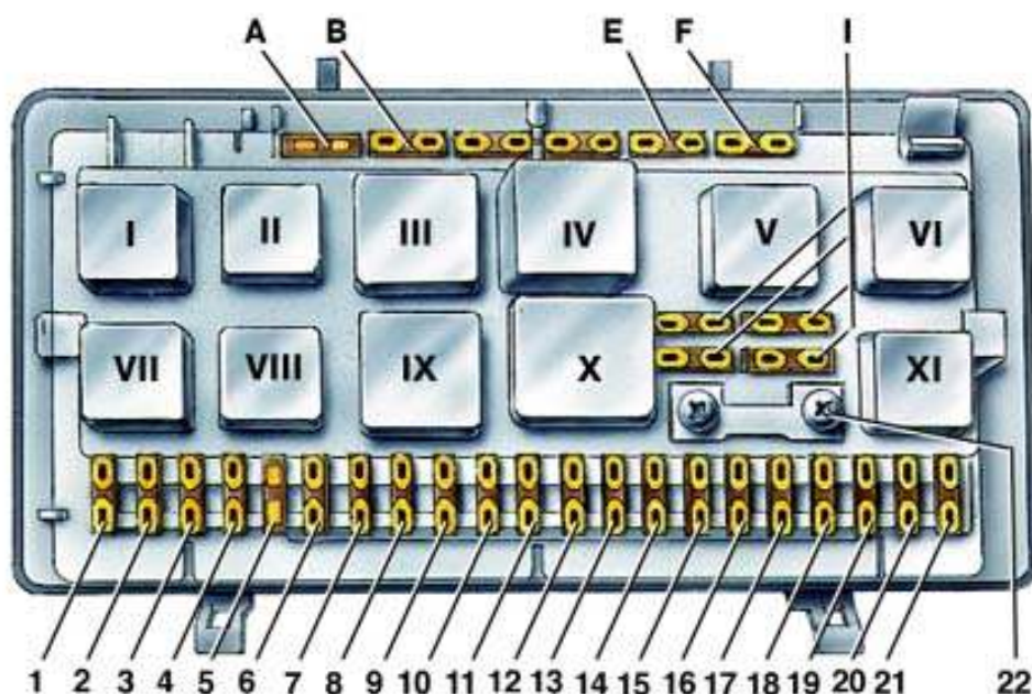
Блок реле и предохранителей
